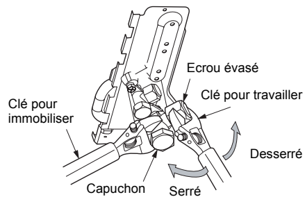
Soupape sur le côté gaz
